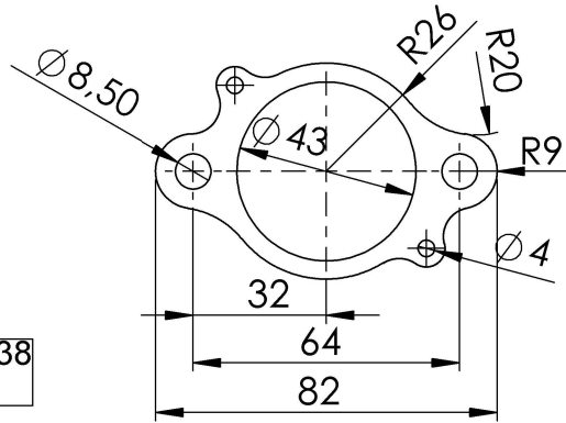
4 S.S. flange Cod."150A"
